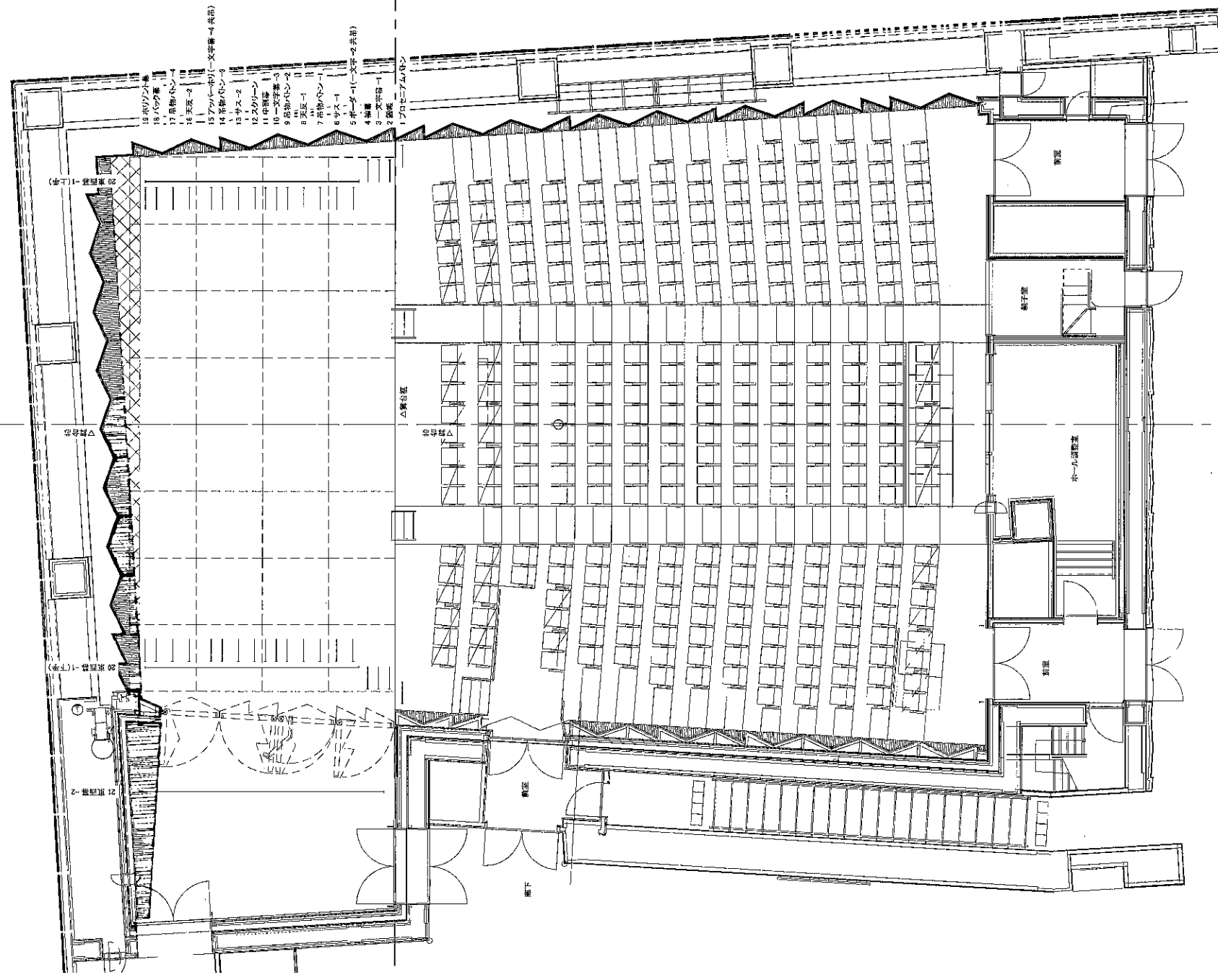
シビックセンターホール ホール平面図 S=1:100 (A3)
